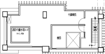
屋突二層平面圖
